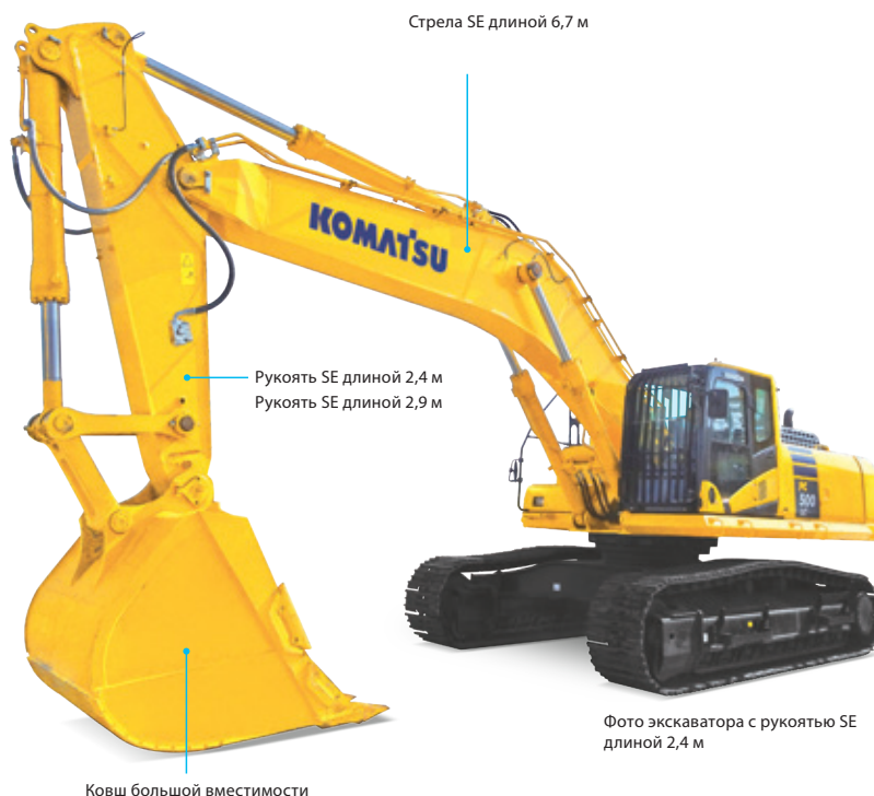
Ковш большой вместимости
